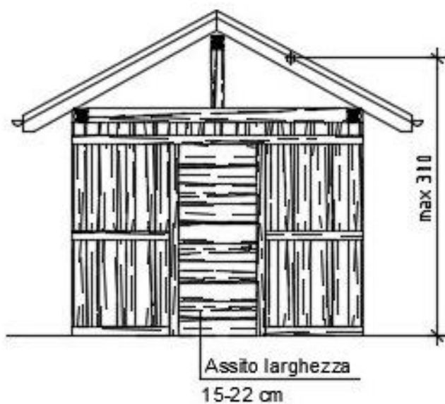
VISTA FRONTALE
