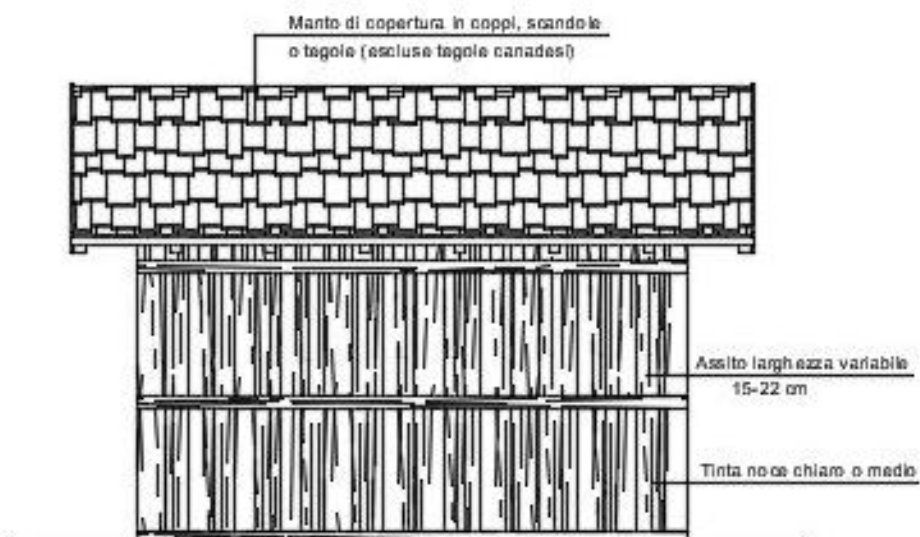
VISTA LATERALE
